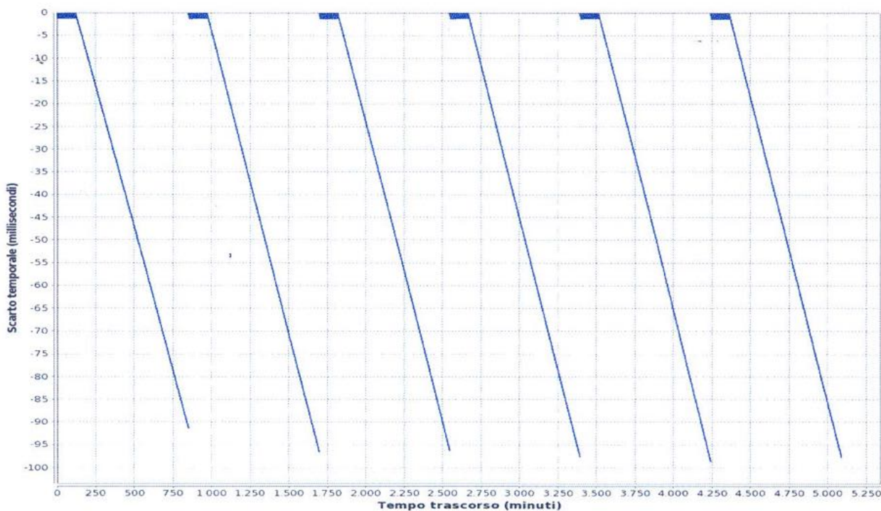
Figura 2 - Andamento dello scarto di tempo nella fase di verifica del funzionamento in assenza di sincronizzazione
