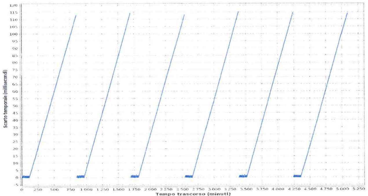
Figura 2 - Andamento dello scarto di tempo nella fase di verifica del funzionamento in assenza di sincronizzazione
